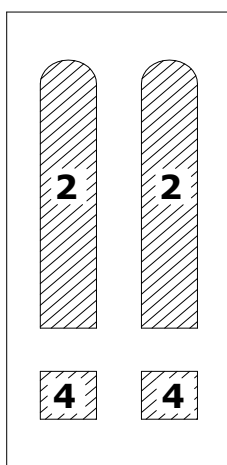
Nílus
