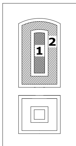
Odera
