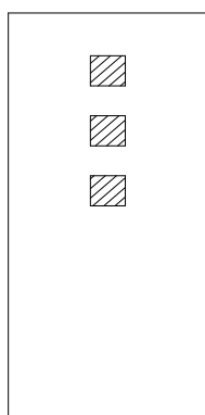
Mars
