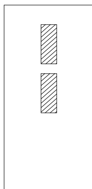
Jupiter
