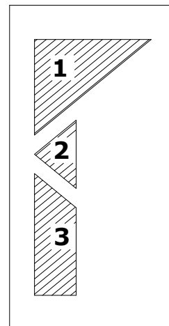
Visztula
