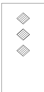
Merkúr
