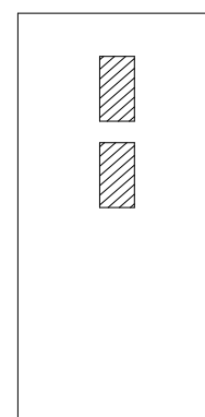
Metis
