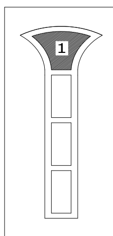
Szamos
