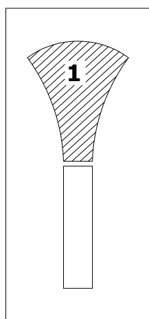
Amazonas
