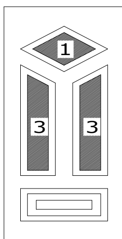
Léna
