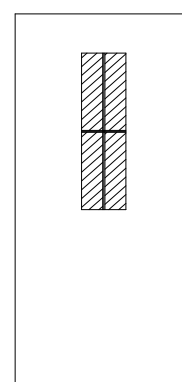
Vénusz
